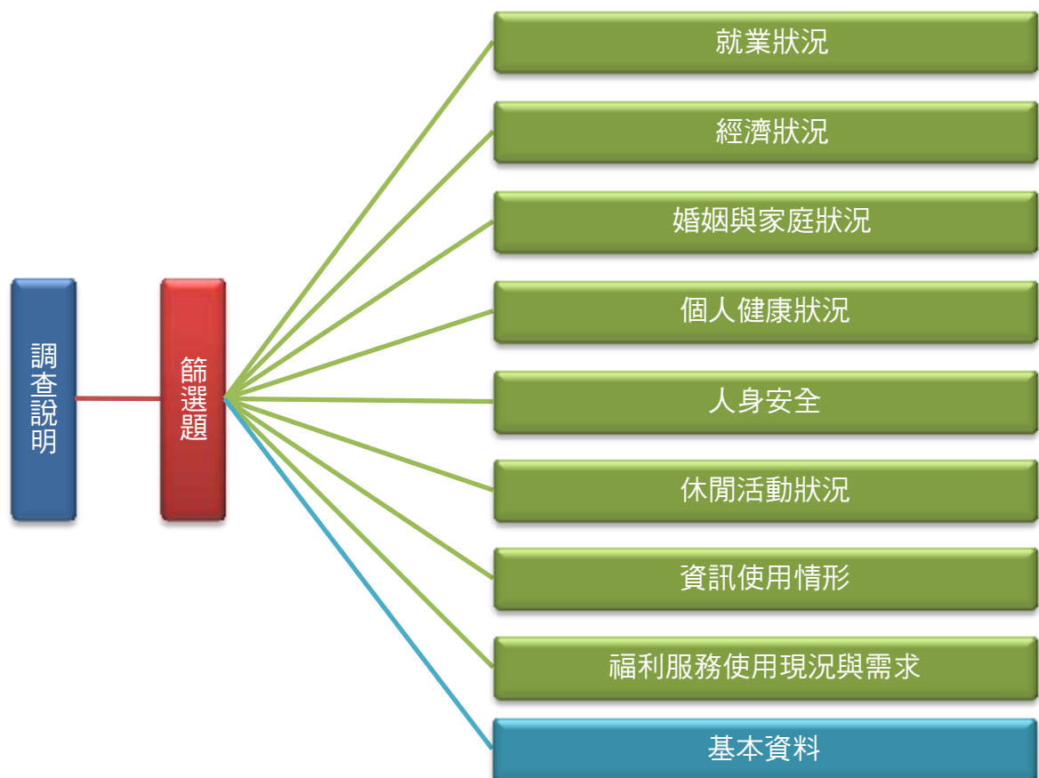
圖 3-1 問卷架構
